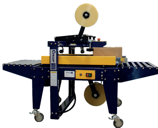
CT 102 mit Förderbändern und Lenkrollen
